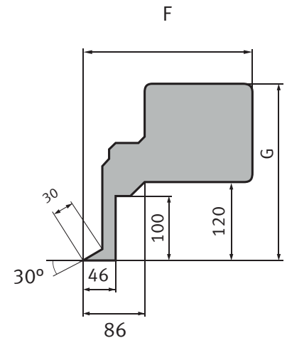
Dimensions tabliers MSBM - SH
