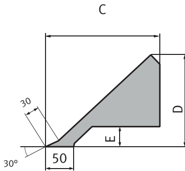
Dimensions tabliers MSBM
