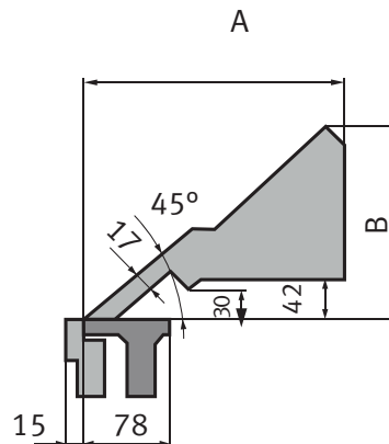
Dimensions tabliers MSBM - S
