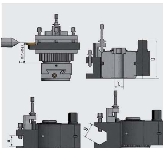
Fig. : Dimensions du corps de tourelle
