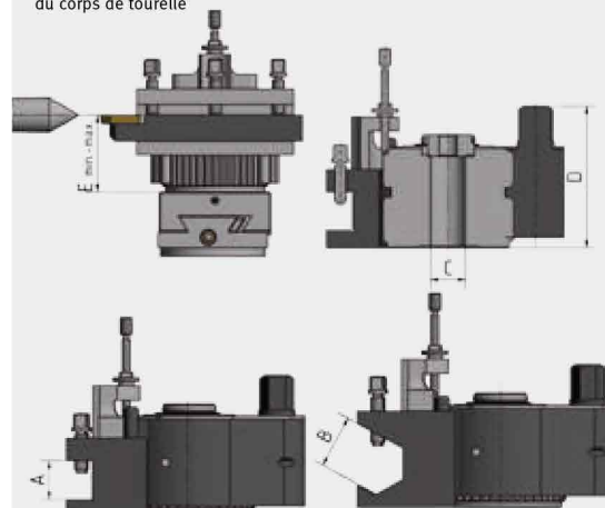
Dimensions du corps de tourelle
